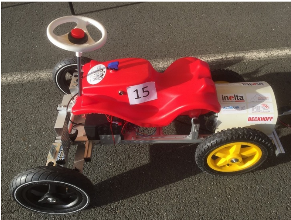
Bild 1: Der modifizierte Solar-Racer: Einzige Bedingung für die Konstruktionsteams war der Erhalt der charakteristischen Karosserie mit Original-Lenkrad und Hupe.
